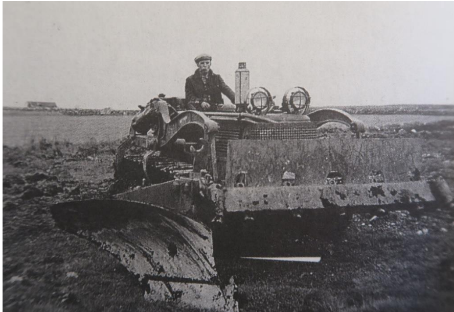
Skjerpeplogen som vart brukt til nydyrking etter krigen. Foto: ukjent.
